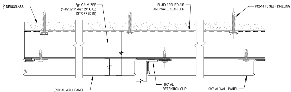
1 HORIZONTAL SECTION Scale: 6"=1'-0"
