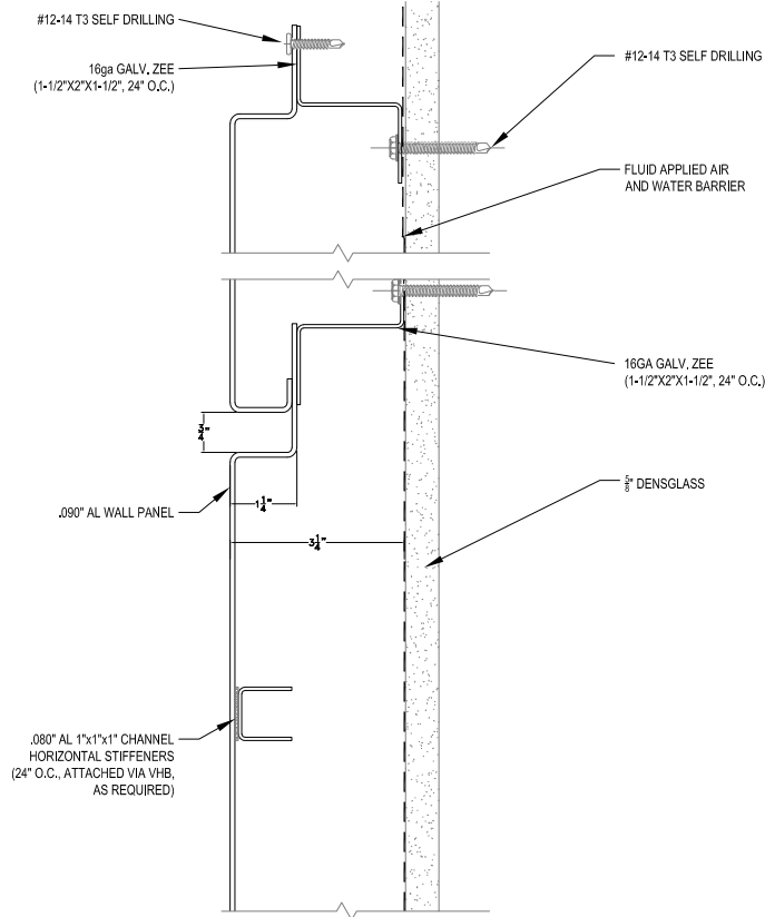
2 VERTICAL SECTION Scale: 6"=1'-0"
